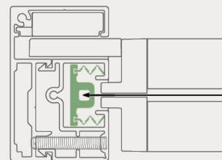
dettaglio Zip
