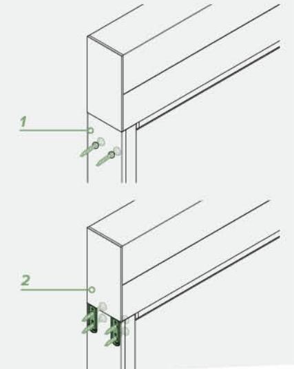
2. fissaggio a spalletta - guide indipendenti
