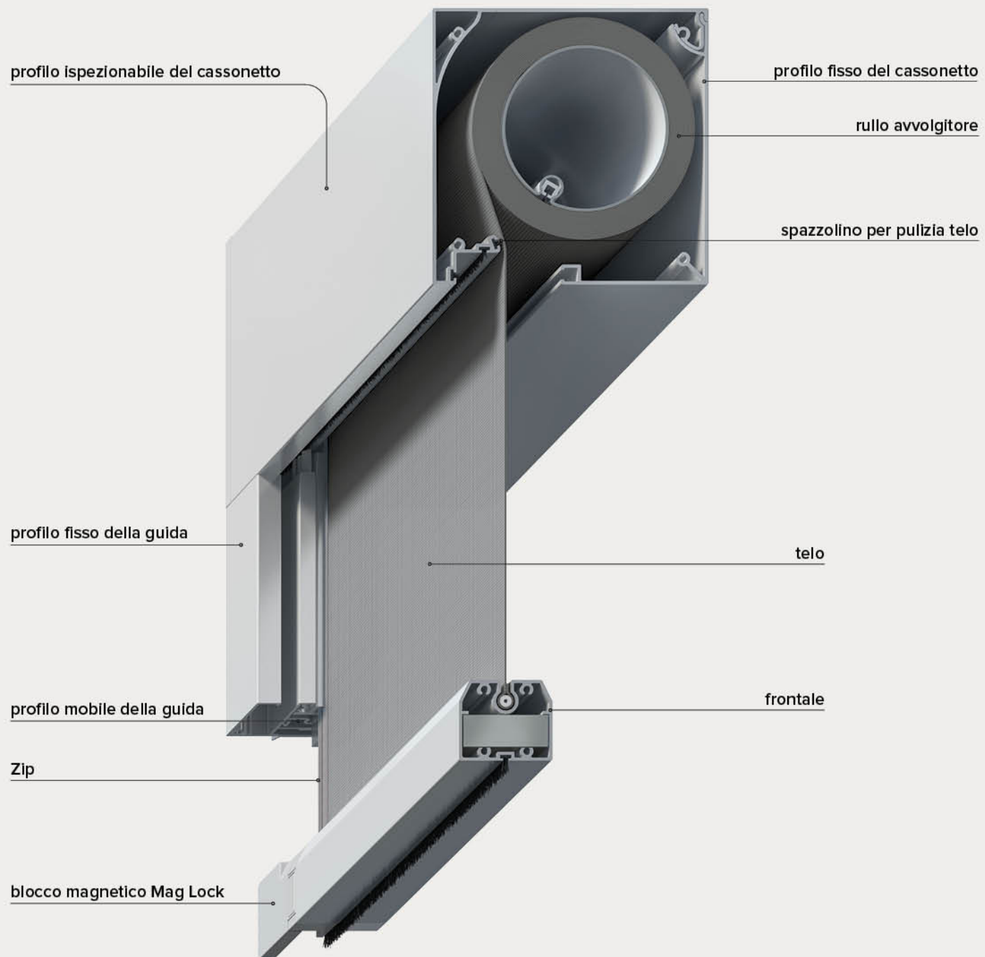
dettaglio Zip
